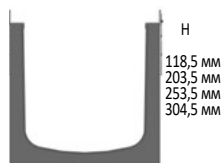
DN200
