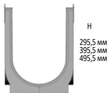
DN300
