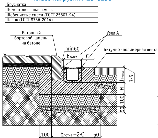
Схема установки пластикового лотка у бордюрного камня класс нагрузки A15-C250
