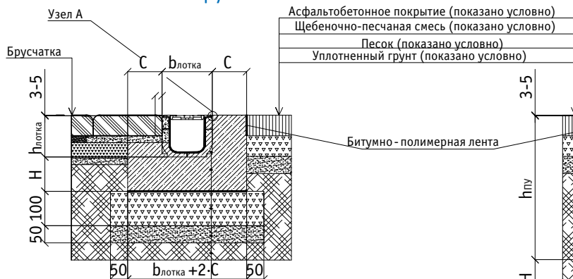
Схема установки пластикового лотка в брусчатое/асфальтобетонное покрытие класс нагрузки A15-C250
